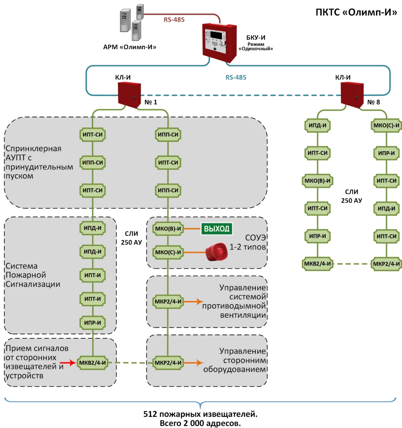
Рисунок 1 – Одиночная система ПКТС (с одним БКУ-И), количество АУ – до 2 000, из них 512 * ИП.
