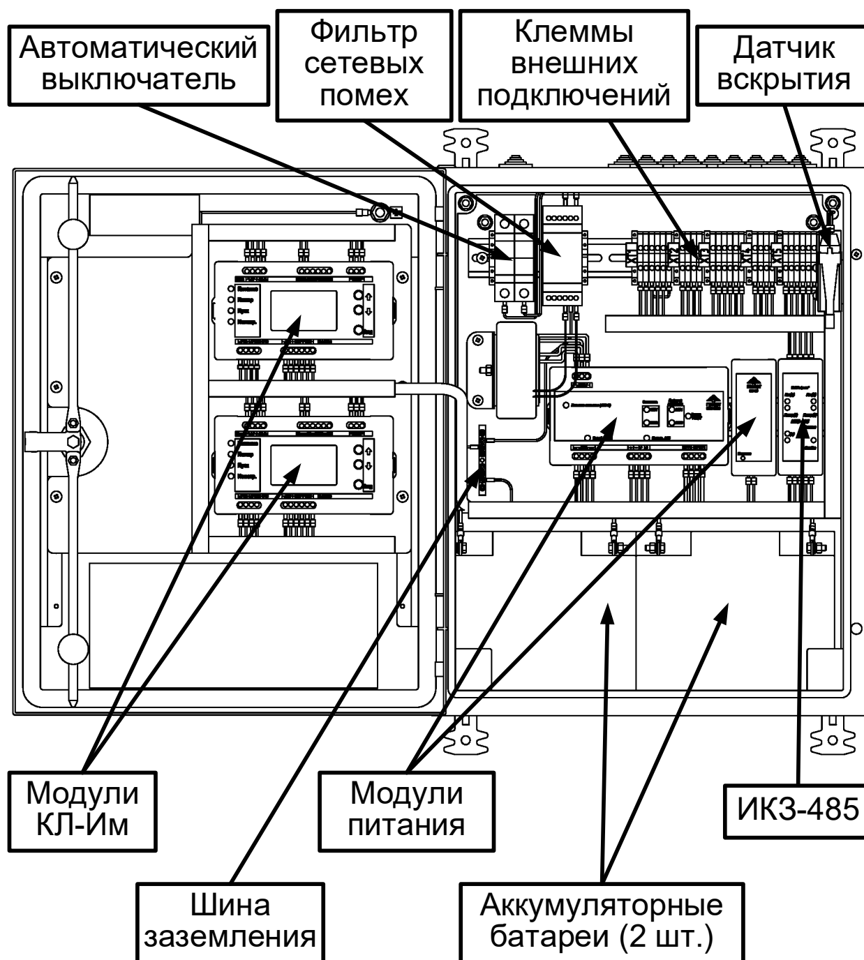
Рисунок 116 – Внешний вид КЛ-И-2 с открытой крышкой.
