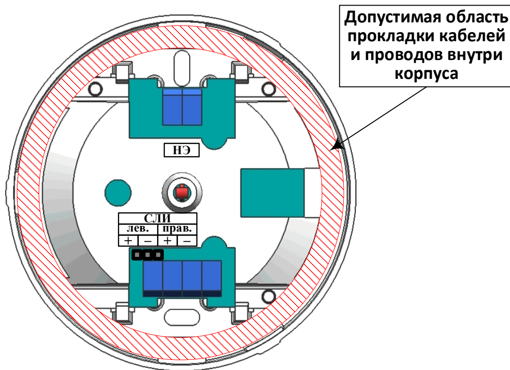
Рисунок 121 – Области прокладки кабелей (проводов) внутри ИПТ-СИ-л, ИПТ-И-л, МКС-И-л.
