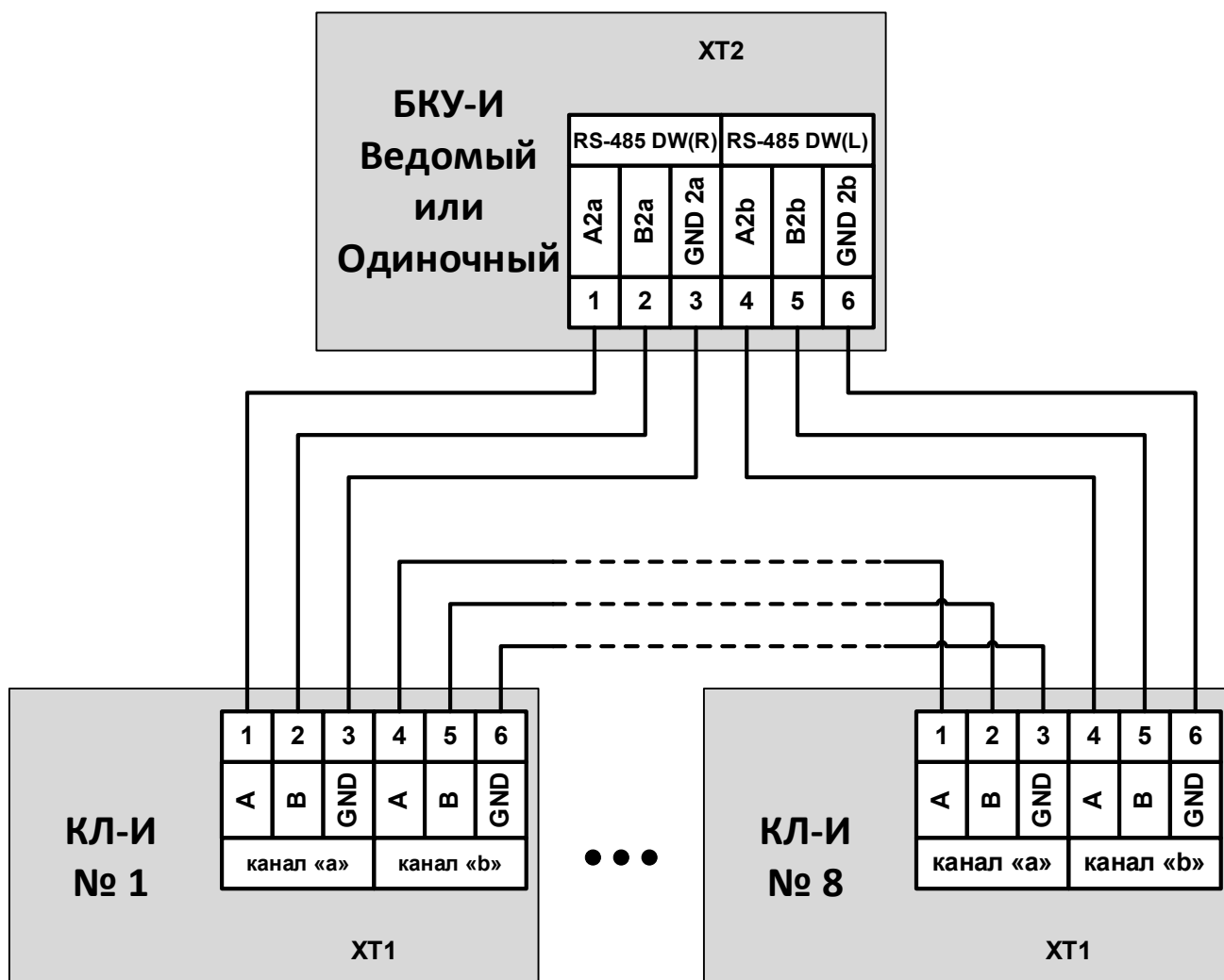
Рисунок 38 – Подключение к БКУ-И кольцевой линии с КЛ-И, КЛ-И-2.
