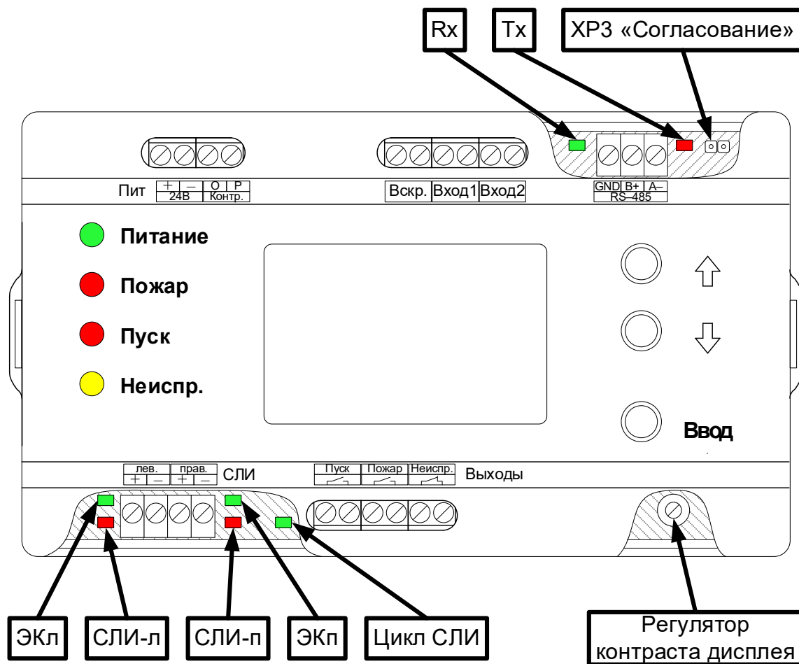
Рисунок 42 – Внешний вид модуля КЛ-Им.
