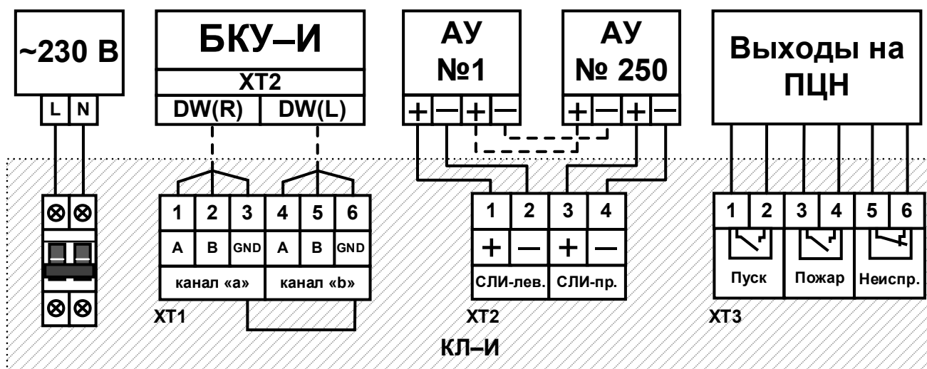
Рисунок 43 – Схема подключений КЛ-И.
