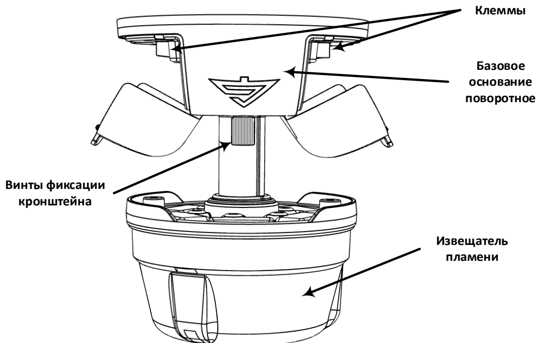
Рисунок 131 – Внешний вид ИПП-СИ.
