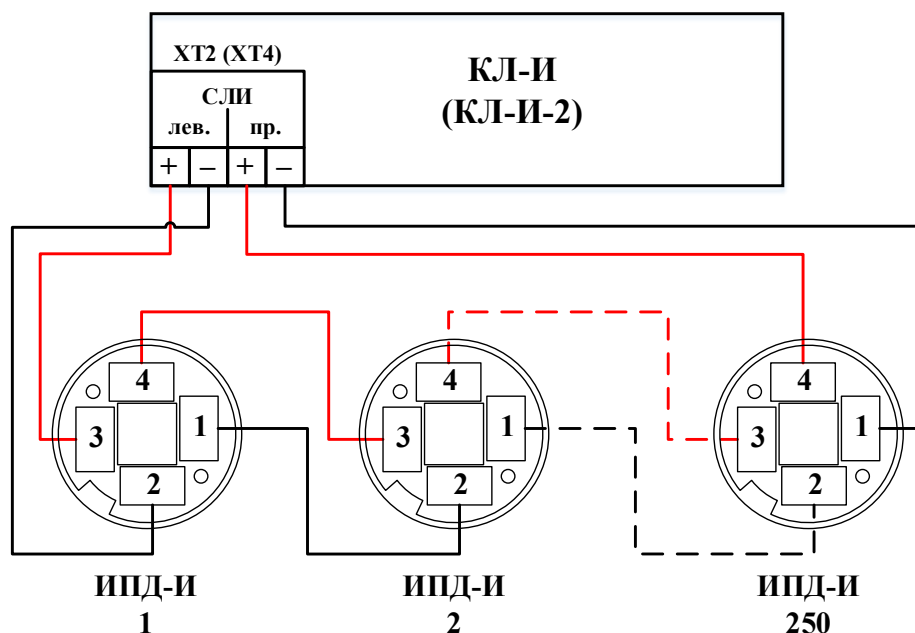
Рисунок 130 – Схема подключения ИПД-И к КЛ-И (КЛ-И-2).
