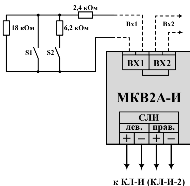
Рисунок 147 – Схема подключения внешних цепей к МКВ2А-И.
