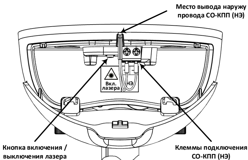
Рисунок 134 – Подключение НЭ СО-КПП.
