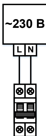
Рисунок 35 – Подключение сети электропитания к БКУ-И.
