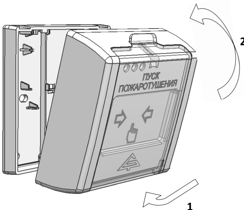
Рисунок 139 – Установка ИПР-И, УДП-И.
