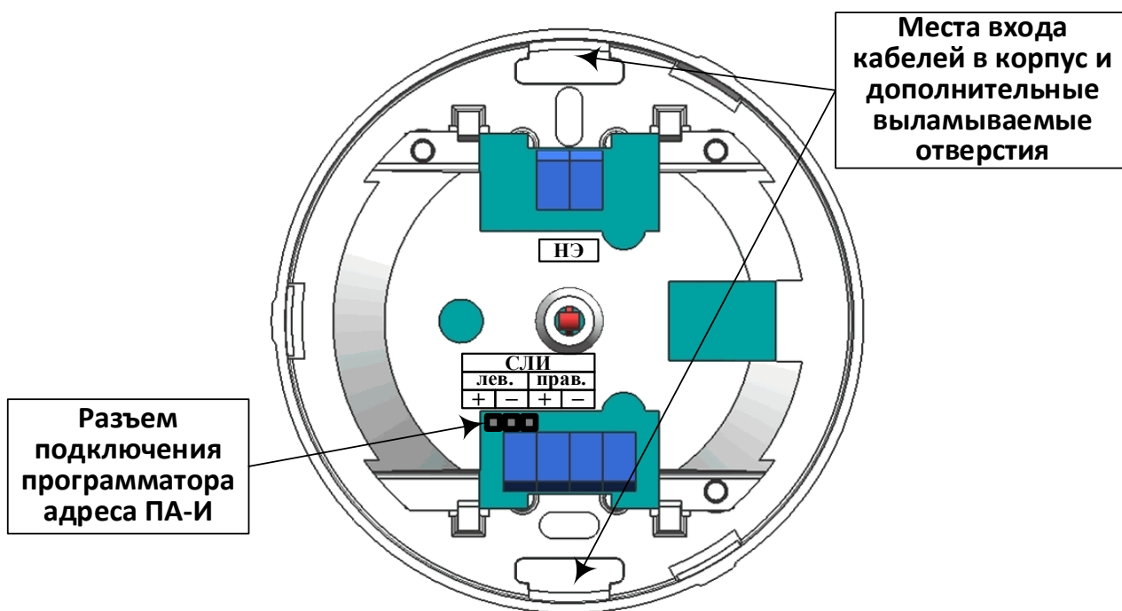
Рисунок 120 – Клеммы подключения внешних цепей к ИПТ-СИ-л, ИПТ-И-л, МКС-И-л.
