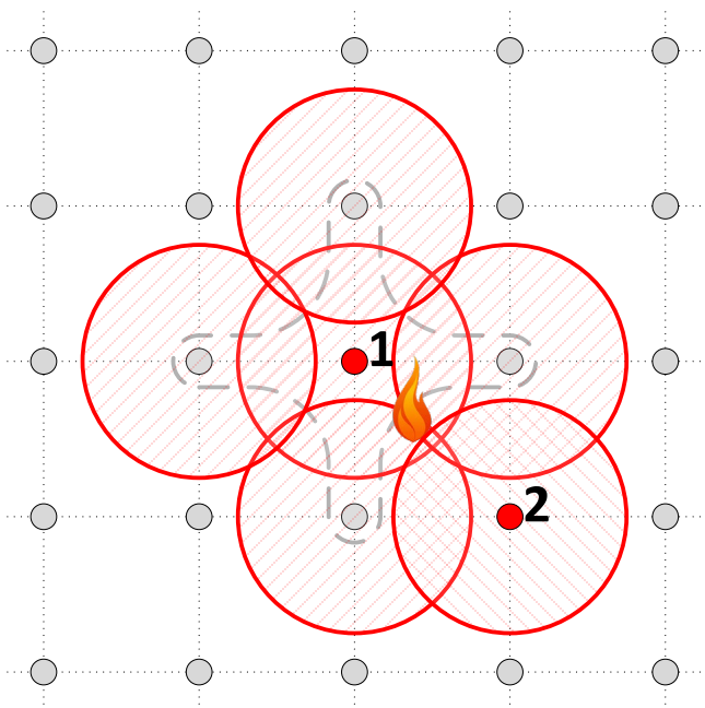
Рисунок 150 – Примеры запуска СО-КПП при наличии у каждого ИП 4 привязок (определяется взаимным расположением сработавших ИП).
