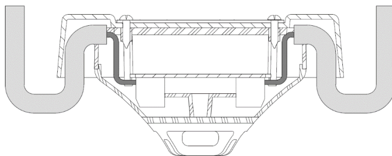
Рисунок 125 – Ввод кабеля под кронштейн.
