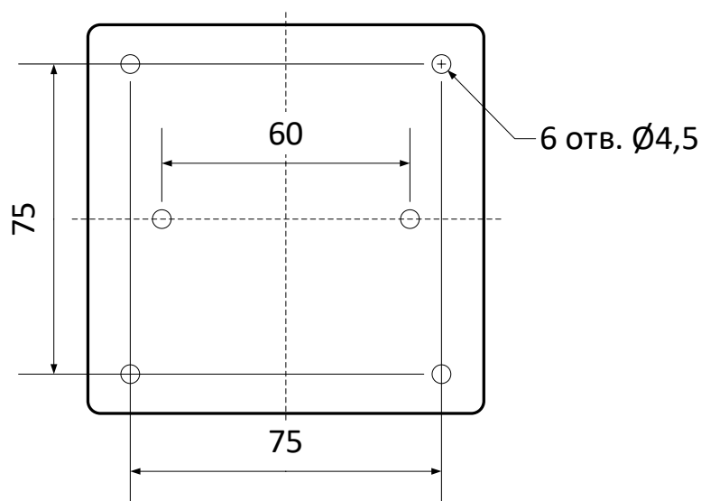
Рисунок 138 – Установочные размеры ИПР-И, УДП-И.
