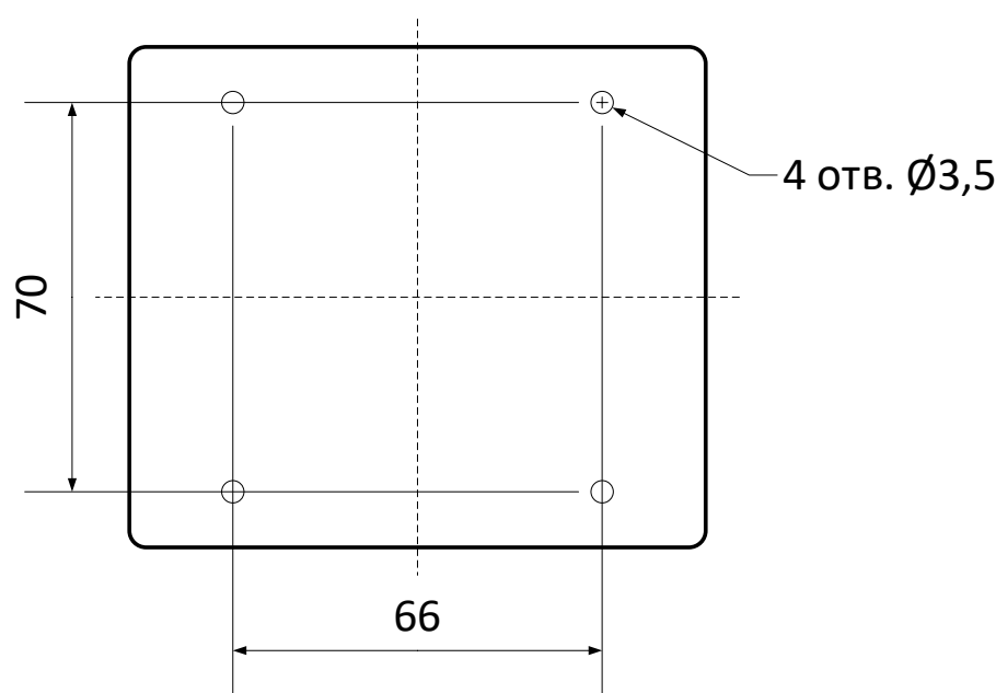
Рисунок 144 – Установочные размеры модулей МКО.
