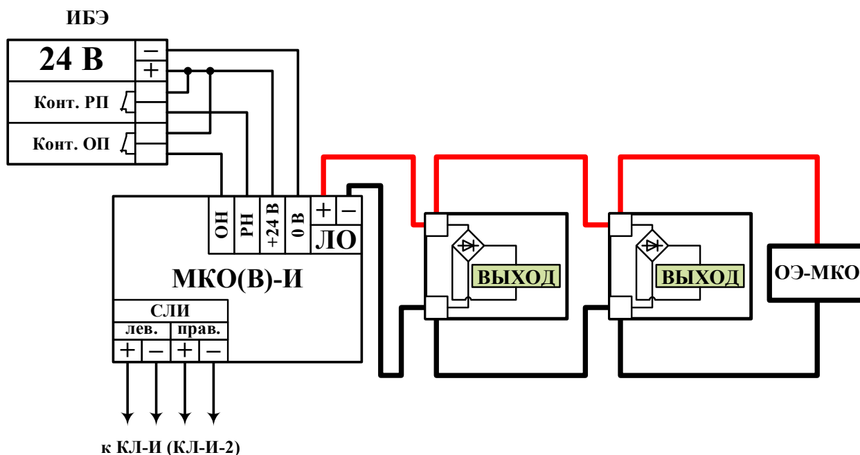
Рисунок 143 – Схема подключения оповещателей к МКО(В)-И. ИБЭ с релейными выходами исправности входов электроснабжения.
