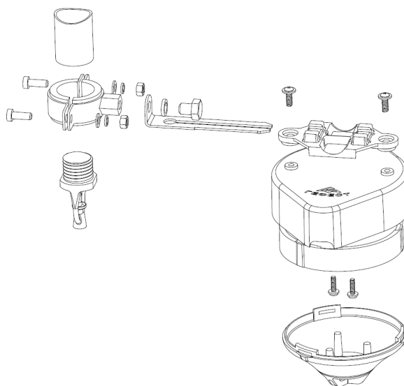
Рисунок 124 – Схема установки ИПТ-СИ-л и МКС-И-л на кронштейн.
