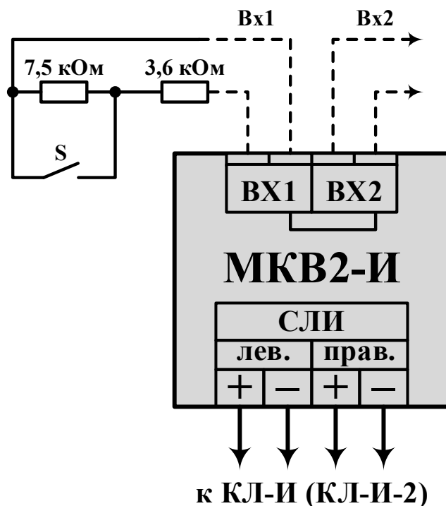
Рисунок 146 – Схема подключения внешних цепей к модулям контроля входов (на примере МКВ2-И).
