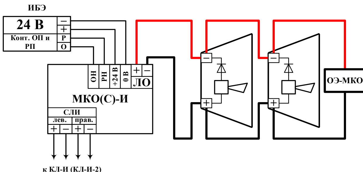
Рисунок 142 – Схема подключения оповещателей к МКО(С)-И.
