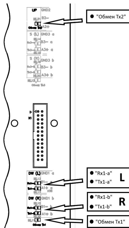
Рисунок 9 – Внутренние светодиодные индикаторы БКУ-И
