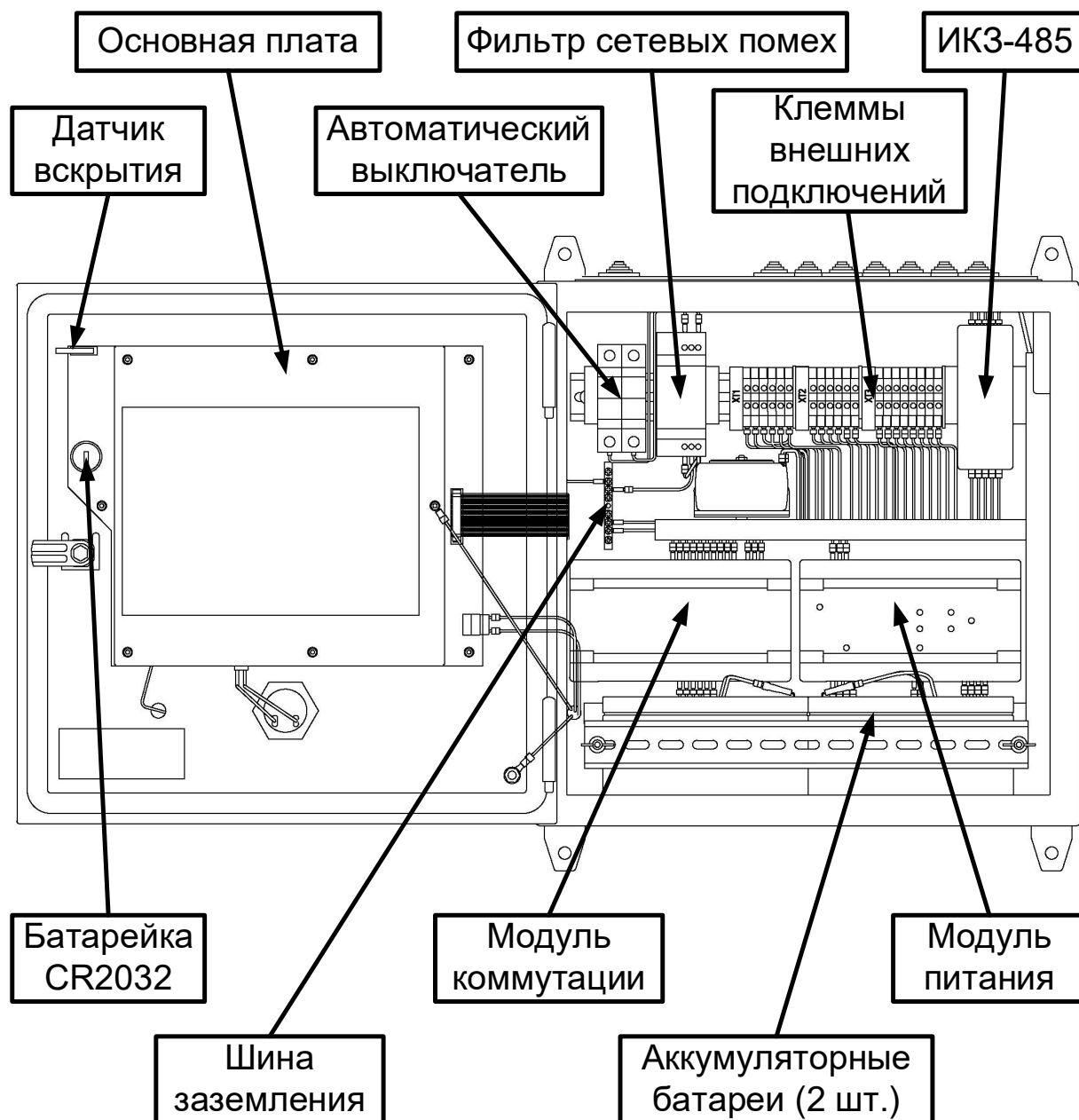
Рисунок 5 – Вид БКУ-И с открытой внешней крышкой.
