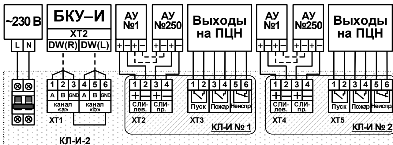
Рисунок 117 – Схема подключений КЛ-И-2.
