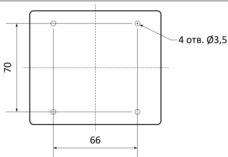
Рисунок 148 – Установочные размеры модулей.
