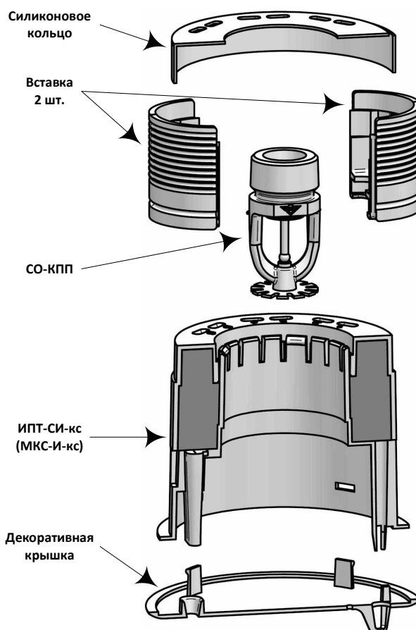
Рисунок 128 – Схема установки ИПТ-СИ-КС и МКС-И-КС на СО-КПП.
