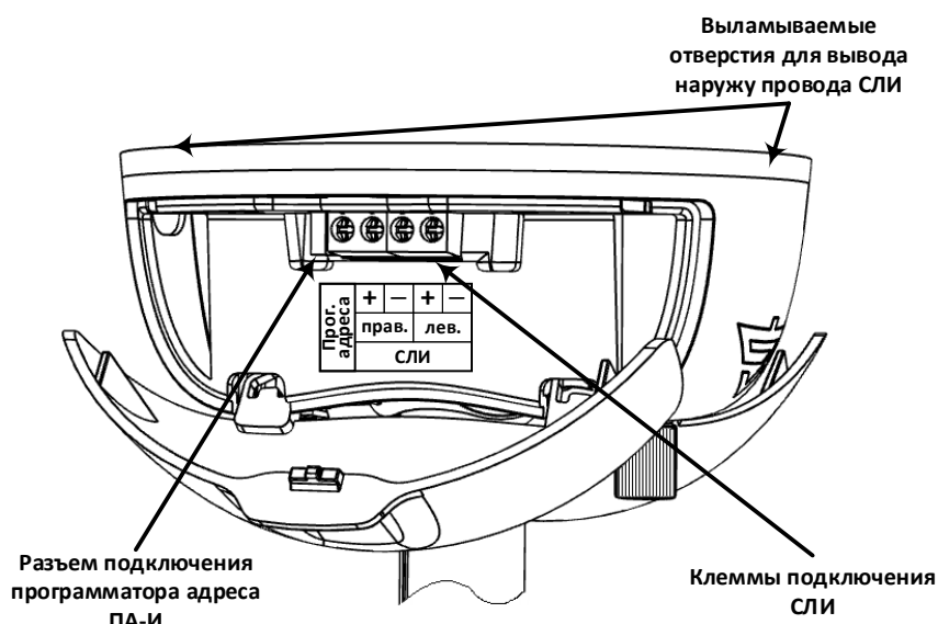
Рисунок 135 – Подключение СЛИ.
