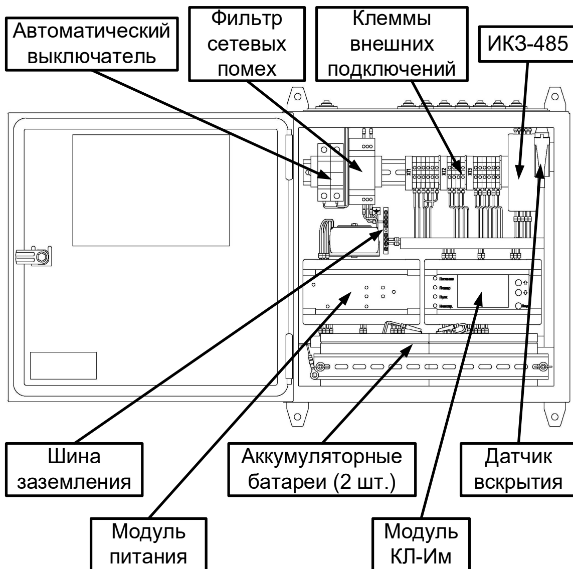
Рисунок 41 – Внешний вид КЛ-И с открытой крышкой.
