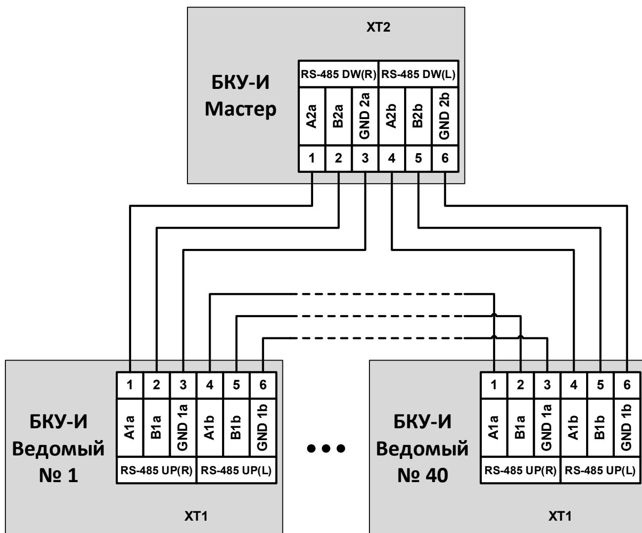
Рисунок 37 – Подключение ведомых БКУ-И к главному БКУ-И–Мастер.
