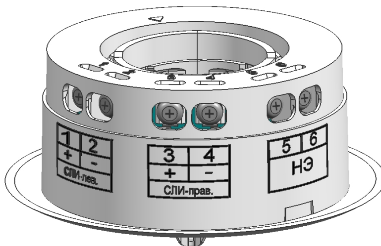
Рисунок 122 – Клеммы подключения внешних цепей к ИПТ-СИ-ку, ИПТ-СИ-кс, МКС-И-ку, МКС-И-кс.
