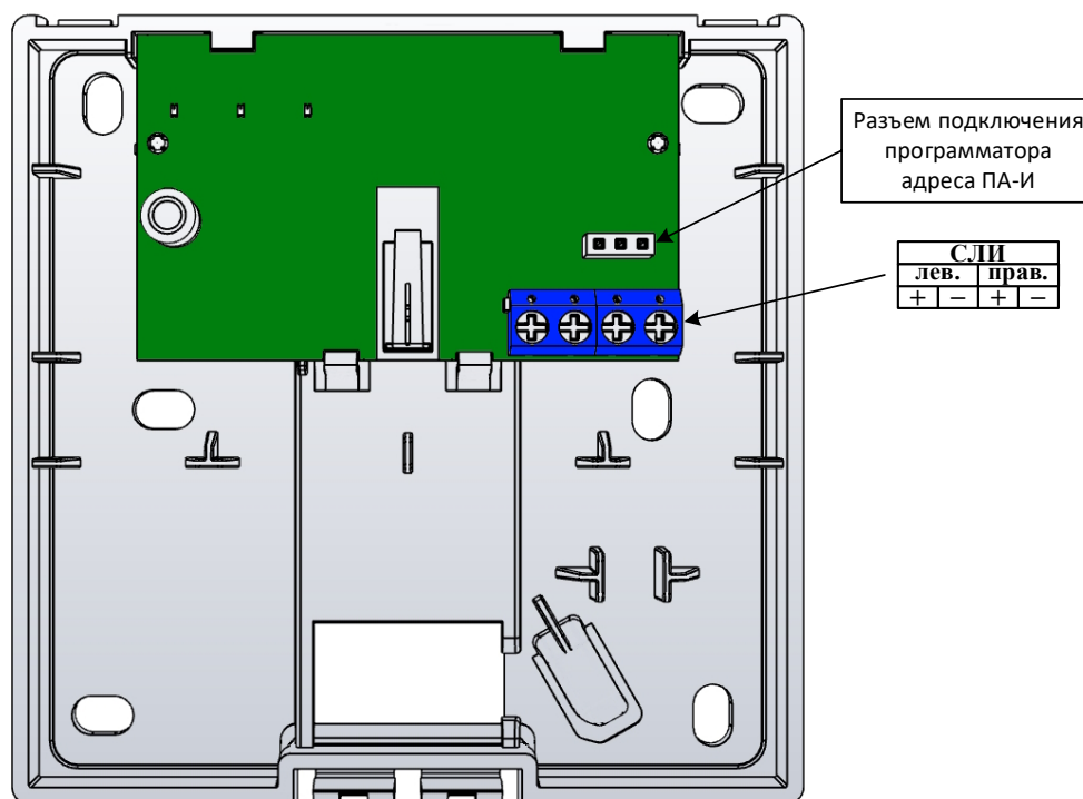
Рисунок 137 – Клеммы подключения внешних цепей к ИПР-И, УДП-И.
