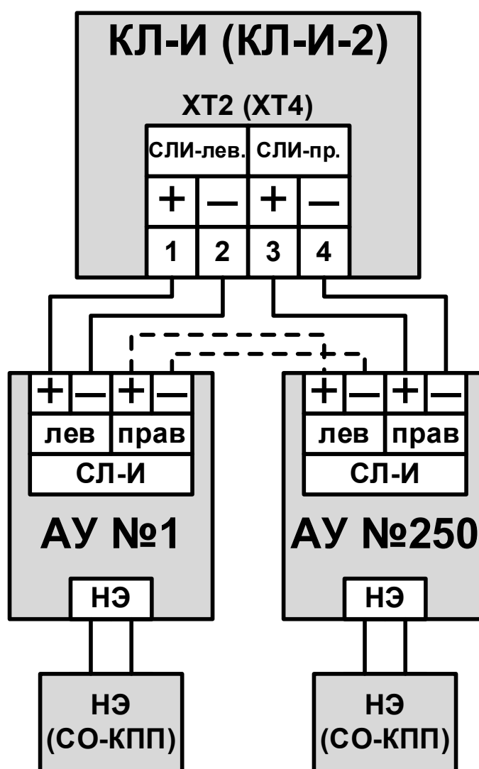
Рисунок 119 – Общая схема подключения АУ к КЛ-И (КЛ-И-2).
