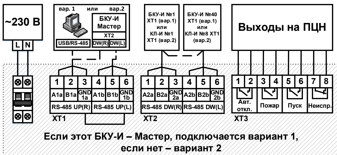
Рисунок 34 – Общая схема подключений БКУ-И.
