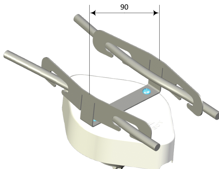
Рисунок 126 – Кронштейн крепления тросовый.
