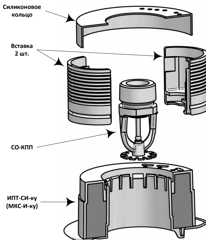
Рисунок 127 – Схема установки ИПТ-СИ-КУ и МКС-И-КУ на СО-КПП.
