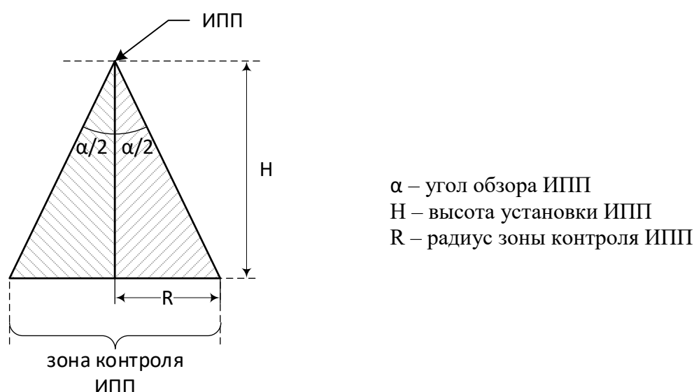
Рисунок 133 – Размер зоны контроля ИПП (вид сбоку).
