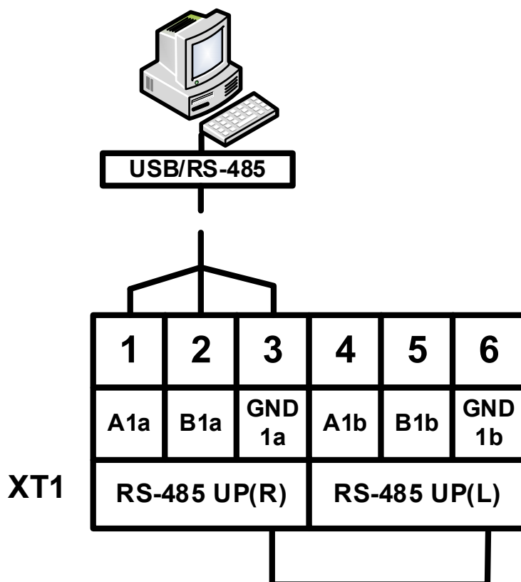
Рисунок 36 – Подключение БКУ-И к компьютеру.
